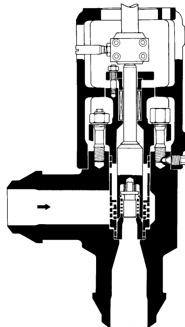
ZK 313-O/13 DN 80-125 mm (3-5")
